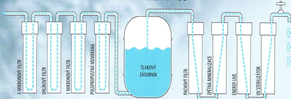
SCHEMA FUNKCE AP-06
